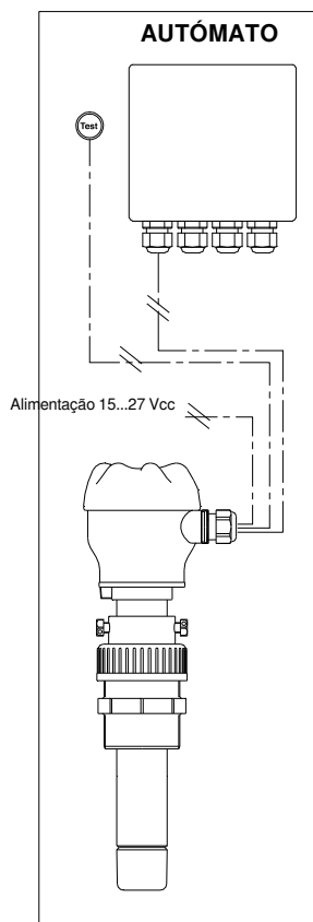
Ligação no autómato
